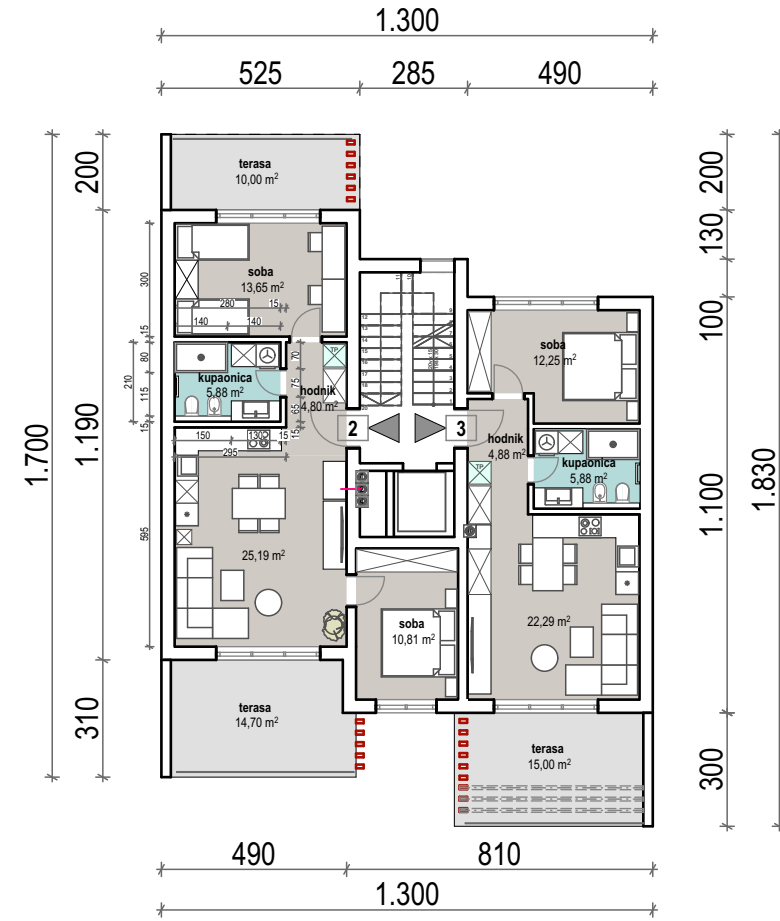
TLOCRT 1.KATA
